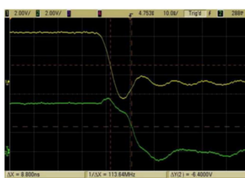
下降沿CKI - CKO延时时间(VCC=5V)
