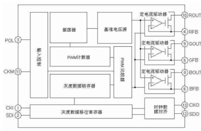
图3：WS2801S集成电路内部功能模块图
