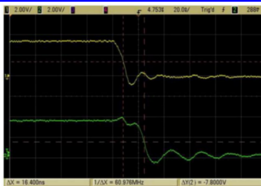
下降沿CKI - CKO延时时间(VCC=3.3V)
