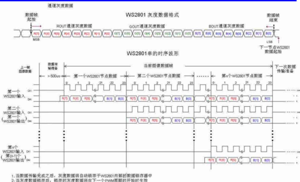
Fig 7. WS2801 的灰度数据格式及时序图
