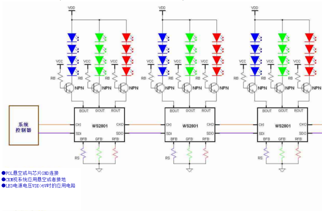
典型应用电路三（使用外部开关实现恒压驱动大功率LED）
