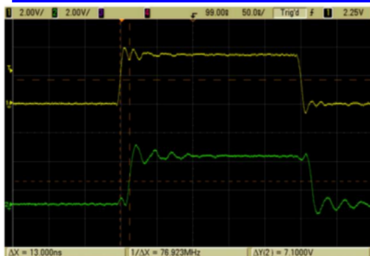
上升沿CKI - CKO延时时间(VCC=3.3V)
