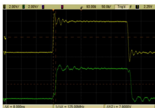
上升沿CKI - CKO延时时间(VCC=5V)
